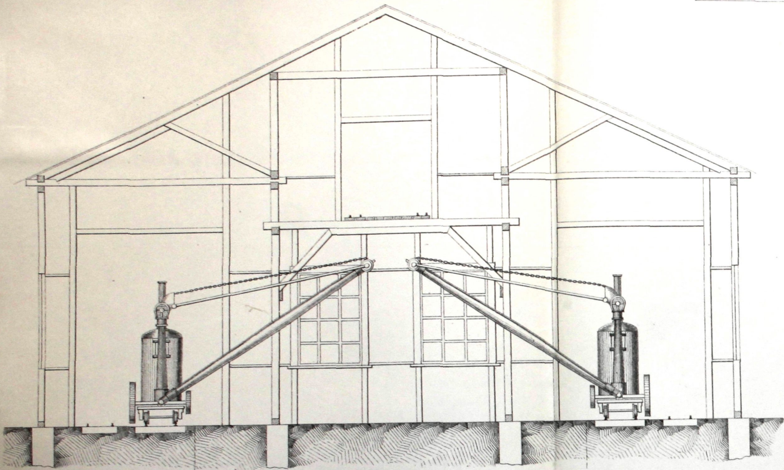
Фиг. 1 bis Схематическій чертежъ расположенія танковъ и экстракторовъ Ванна для газурки хвостовъ. труба труба цилиндръ
