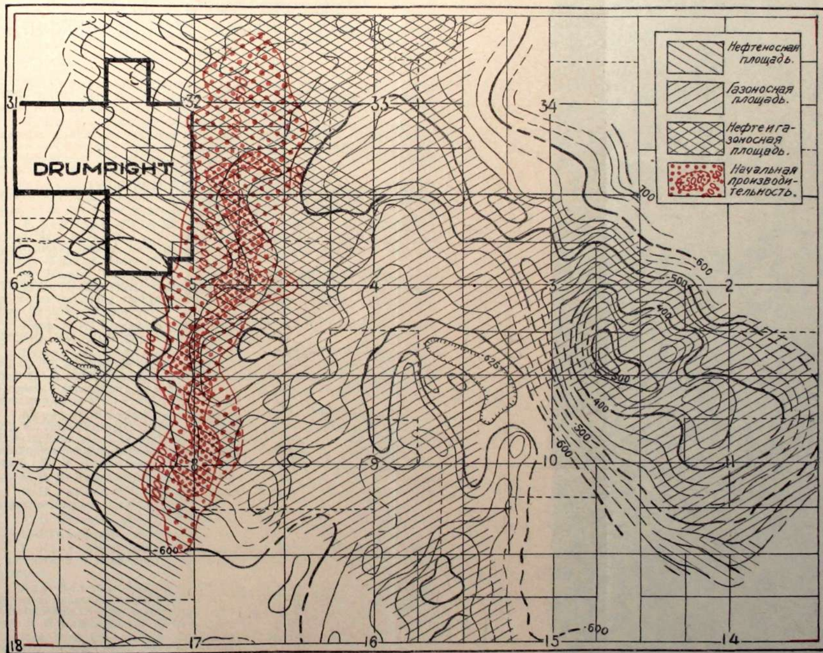
купол ДРЭМРАЙТ на площади КЭШИГ, ОКЛЯХОМЯ. ПОКАЗАНО РАСПОЛОЖЕНИЕ СКВАЖИН НАИВЫСШЕЙ НАЧАЛЬНОЙ ПРОИЗВОДИТЕЛЬНОСТИ.
